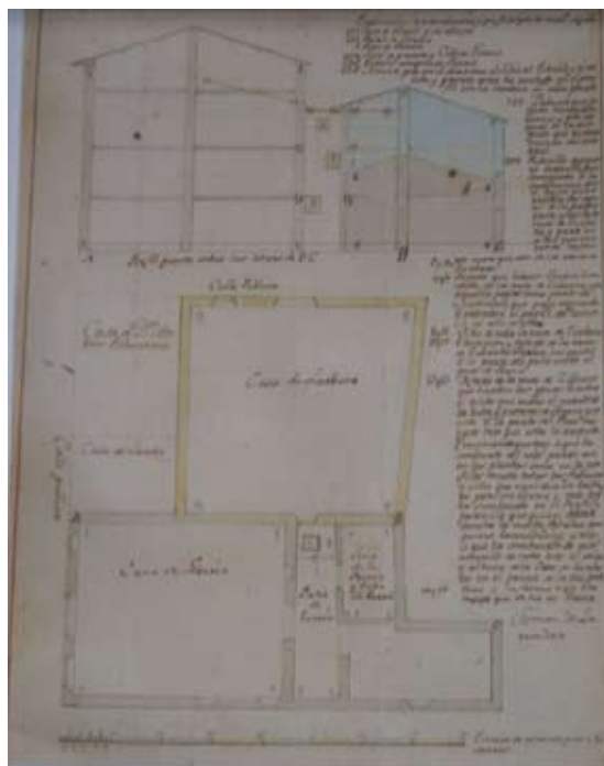
Plano de la casa del un maestro pelaire Pedro Gerónimo Gorri
